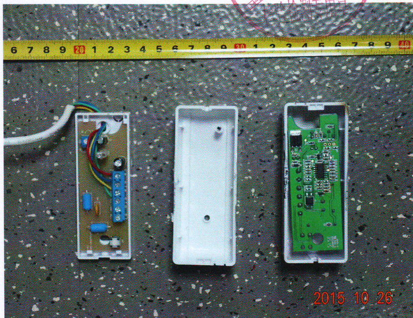
图二、NS-100V 振动入侵探测器内部结构
